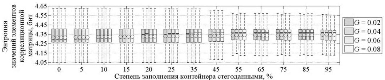
Рисунок 2 – Результаты АСС стеганограм, сформированных согласно методу Дея – энтропия значений элементов КМ
