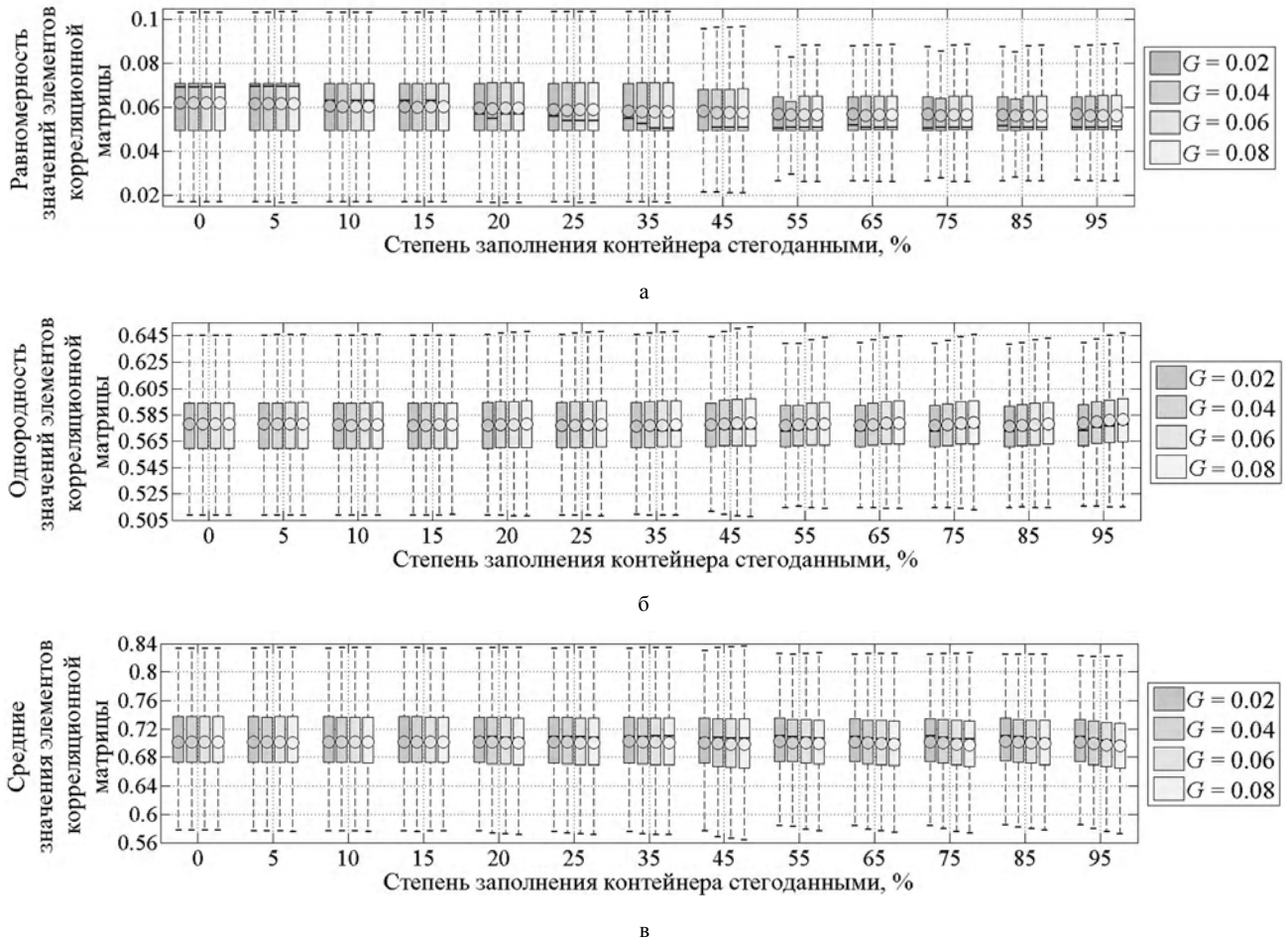
Рисунок 1 – Результаты АСС стеганограм, сформированных согласно методу Дея: а – равномерность значений элементов КМ; б – однородность значений элементов КМ; в – средние значения элементов КМ
